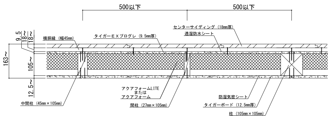
水平断面図
